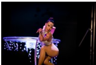
Pierścienie Saturna 2019
