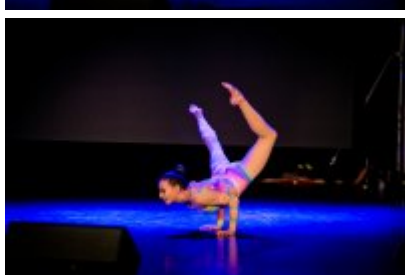
Pierścienie Saturna 2019
