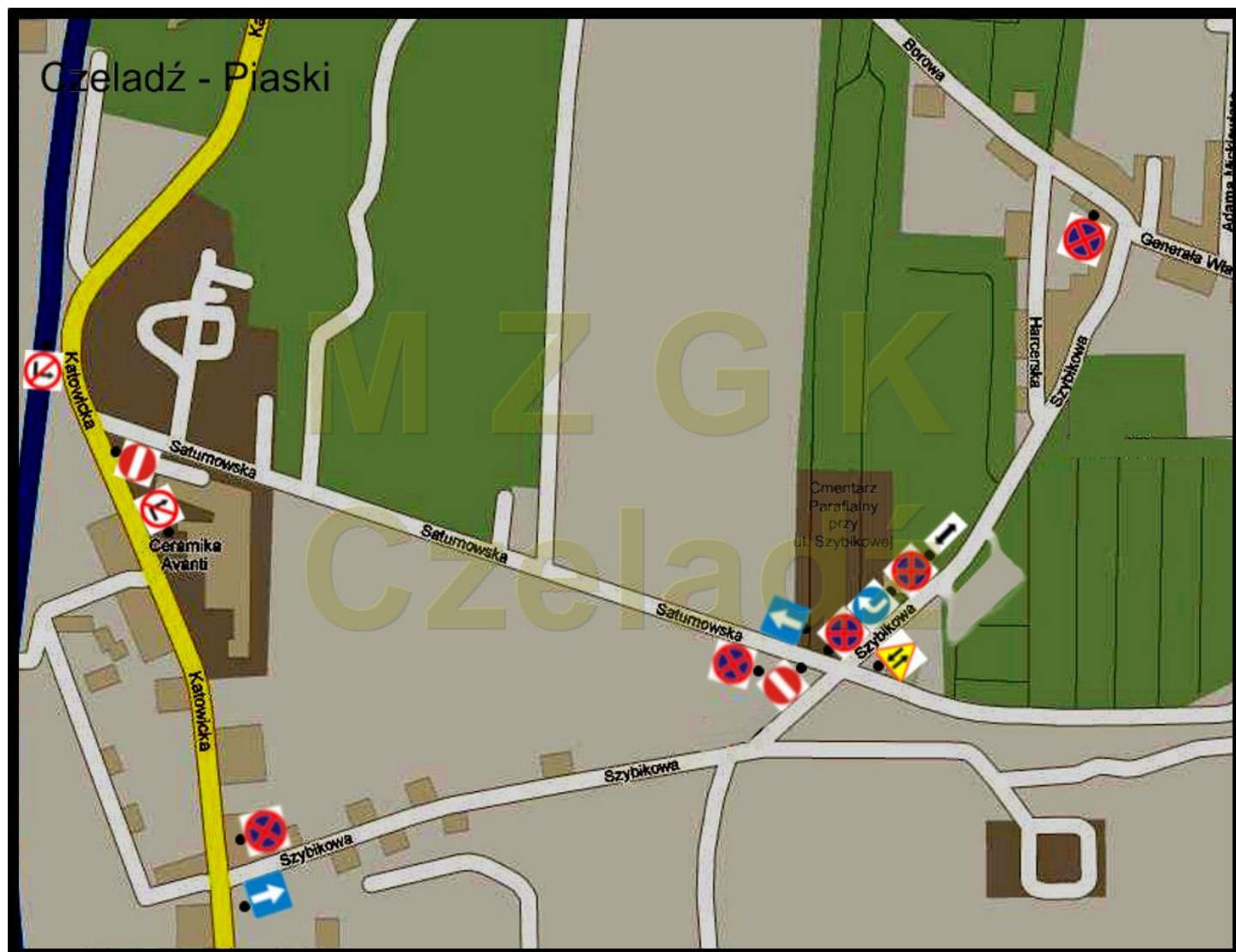
Schemat zmiany organizacji ruchu w pobliżu cmentarza przy ul. Szybikowej
